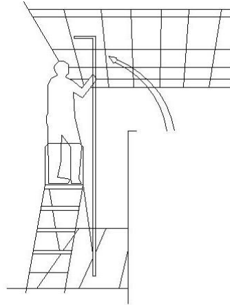
MONTAJE TÍPICO PILAR DE SERVICIO
