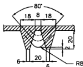
CORTE D-D
